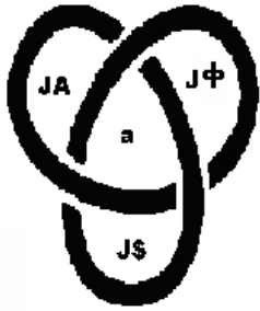
Nœud en trèfle
